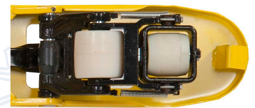
Rodillos de entrada y salida adicionales.
